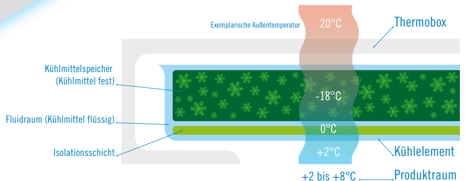
Schnittdarstellung ICECATCH Solid Insulated
